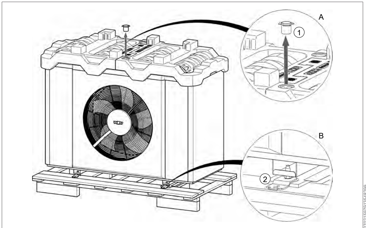
1 Kondensatstutzen
