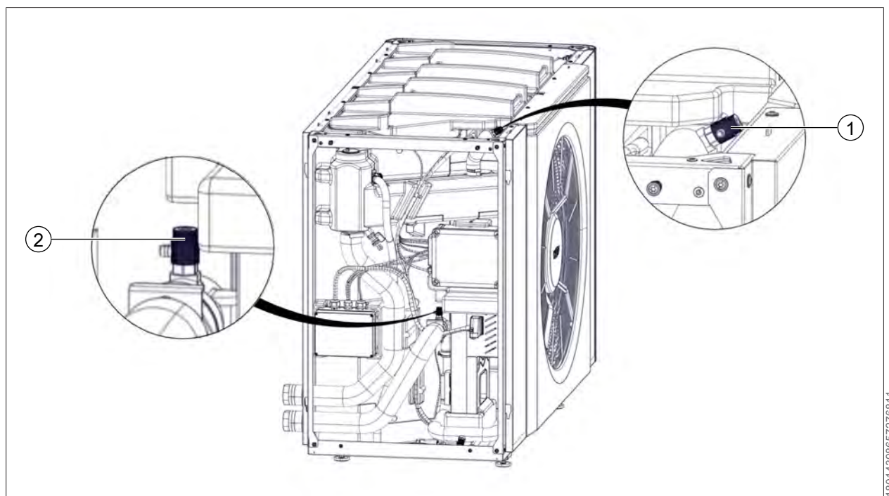
1 Handentlüfter (Luft-/Klätemittelabscheider)
