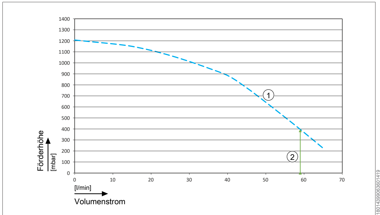
1 Kennlinie CHA-20/24
