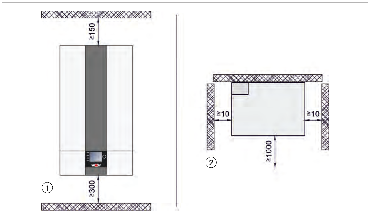
1 Frontansicht IDU
